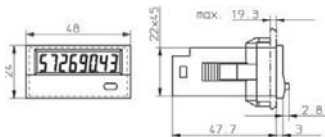
Dimensions CODIX 141 et 143
