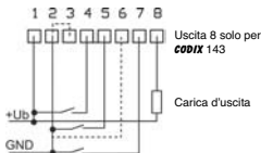
Assegnazione dei morsetti
